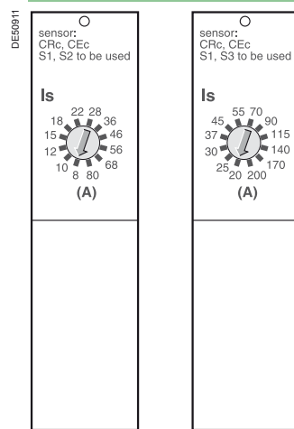
S1-S2 wiring
