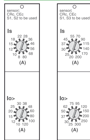
S1-S2 wiring
